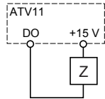
Schema con alimentazione interna:
