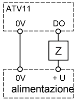
Schema con alimentazione esterna:
