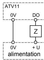
Schéma avec alimentation externe :
