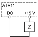
Schéma avec alimentation interne :
